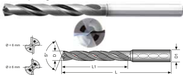
Durch die neue Nutengeometrie entstehen kurze und kompakte Späne.
