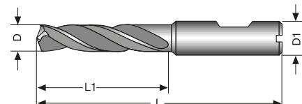
HB mit Kühlkanal
