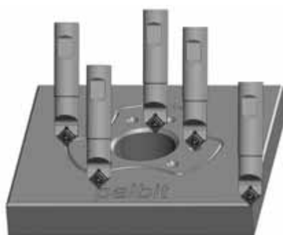
Zentrieren, Fasen, Gravieren
